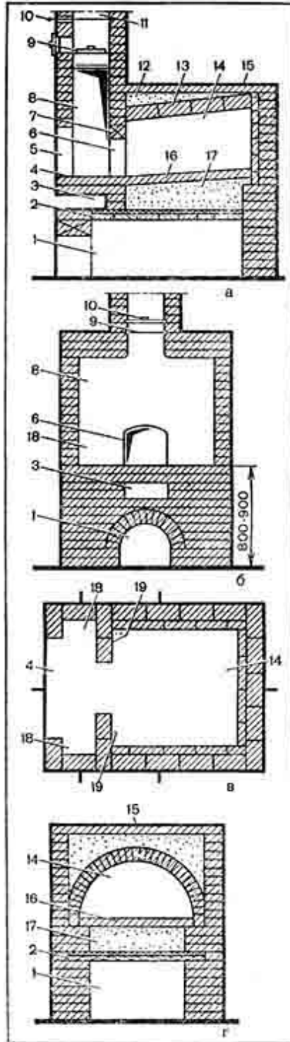
Рис. 67. Детали обыкновенной русской печи:
