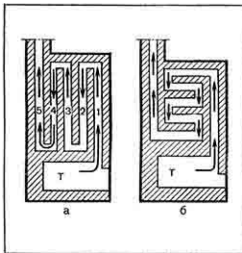
Рис. 45. Многооборотные схемы:
