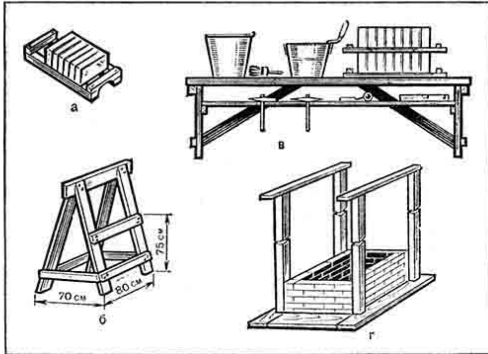
Рис. 12. Приспособления:
