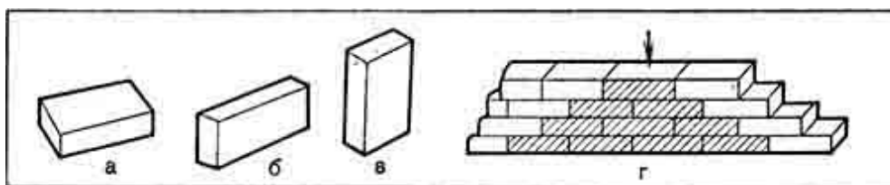
Рис. 17. Укладка кирпича:
