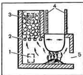
Рис. 110. Банная печь-каменка:
