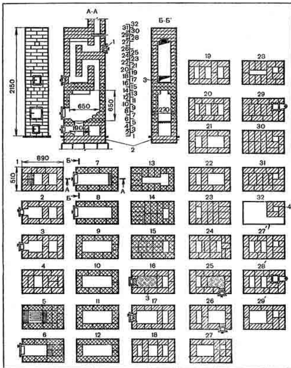
Рис. 75. Отопительная печь, оштукатуренная, с теплоотдачей 1940 ккал/ч:
