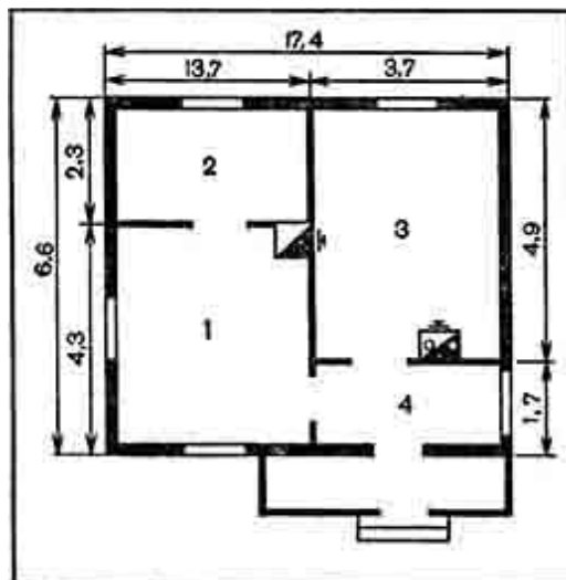
Рис. 22. Установка печей в комнатах дома и их подбор на теплоотдачу:
