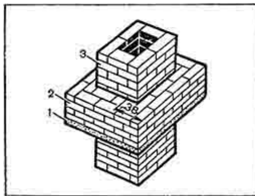
Рис. 101. Железобетонная плита для поддержания кирпичной разделки:
