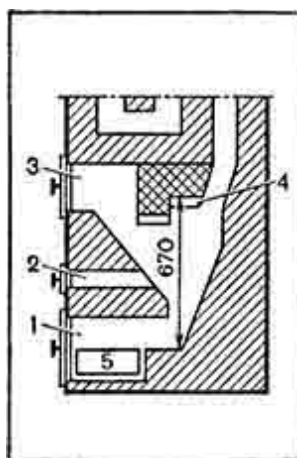
Рис. 39. Топливник для сланцев:
