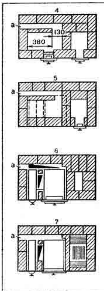
Рис. 53. Варианты отвода дымовых газов с торцевой стороны плиты:
