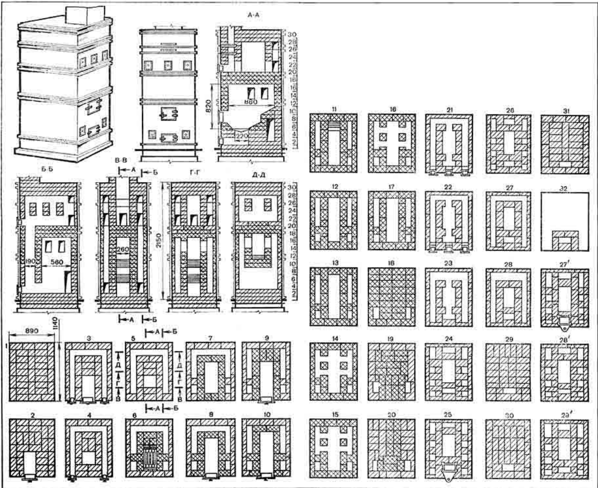
Рис. 79. Отопительная печь в металлическом футляре с теплоотдачей 3920 ккал/ч
