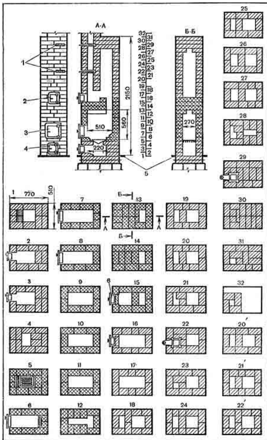
Рис. 74. Оштукатуренная отопительная печь с теплоотдачей 1760 ккал/ч:
