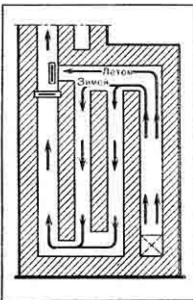
Рис. 57. Отопительный щиток с двумя ходами: зимним и летним
