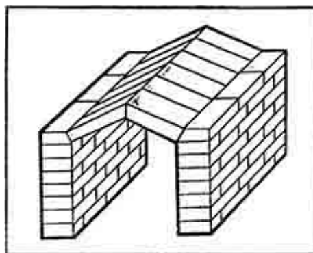
Рис. 27. Перекрытие узкого топливника треугольным сводом
