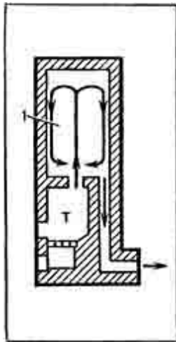
Рис. 46. Бесканальная схема:
