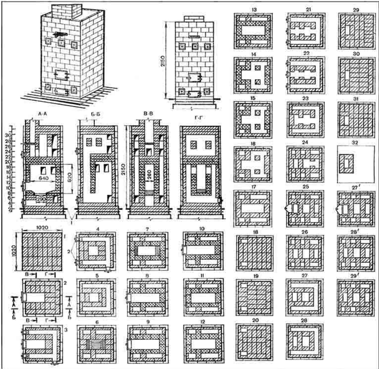
Рис. 80. Отопительная печь изразцовая с теплоотдачей 4150 ккал/ч: 1 — гидроизоляция; 2 — чистки
