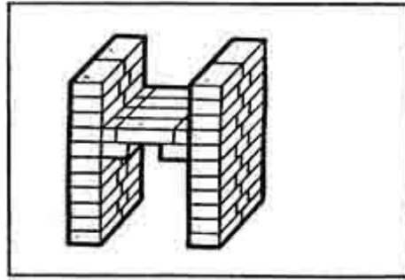
Рис. 29. Перекрытие топливника путем выпуска кирпича из боковых сторон кладки
