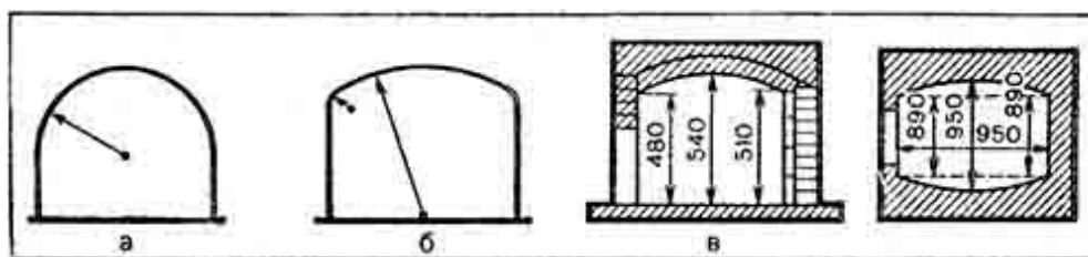
Рис. 68. Форма сводов:
