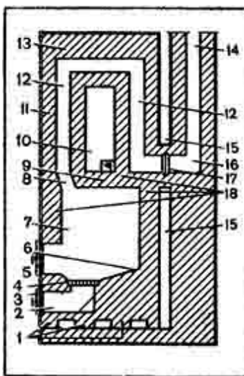
Рис. 37. Схема отопительной печи:
