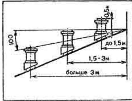
Рис. 84. Расположение труб на крыше
