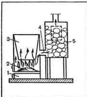
Рис. 114. Печь-каменка из металла:
