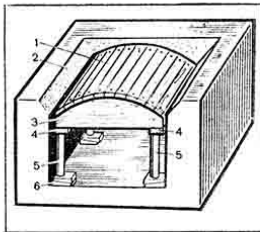
Рис. 33. Опалубка для кладки сводов:
