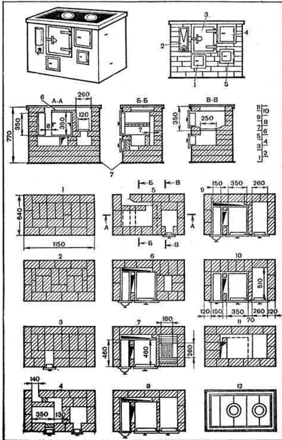
Рис. 52. Кухонная плита с духовкой и водогрейной коробкой:
