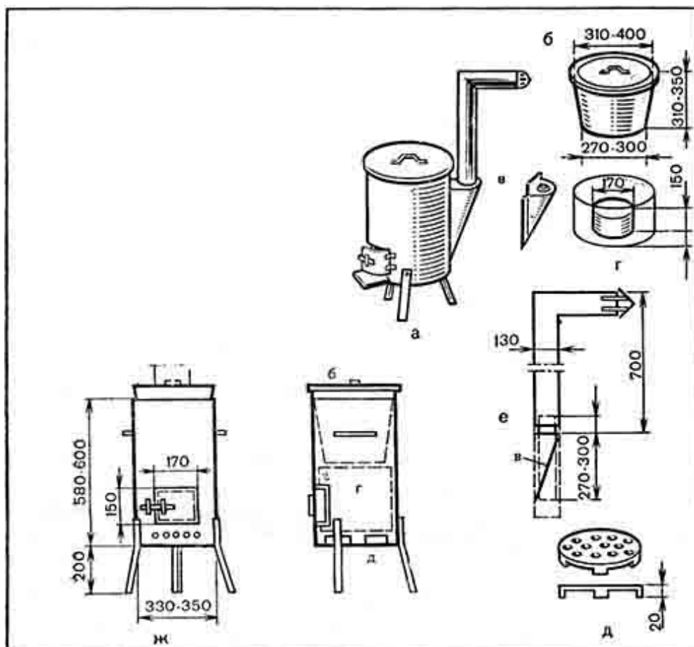
Рис. 115. Печка-прачка:
