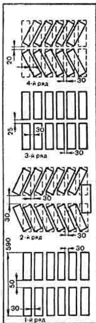
Рис. 4. Схема укладки кирпича для сушки
