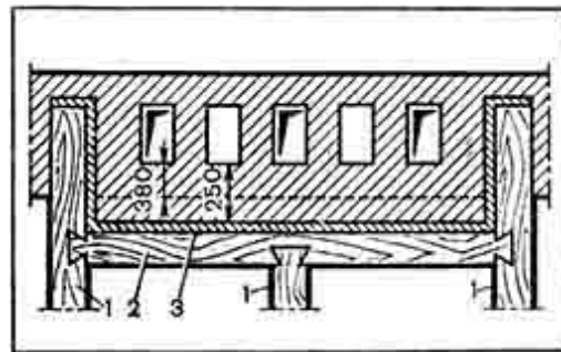
Рис. 99. Устройство ригеля:
