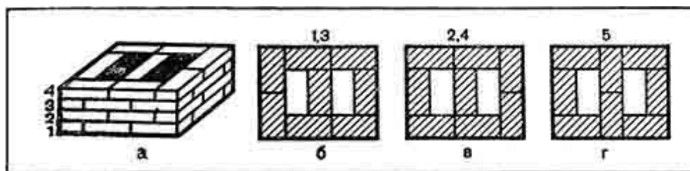
Рис. 86. Кладка трубы при двух спаренных каналах:
