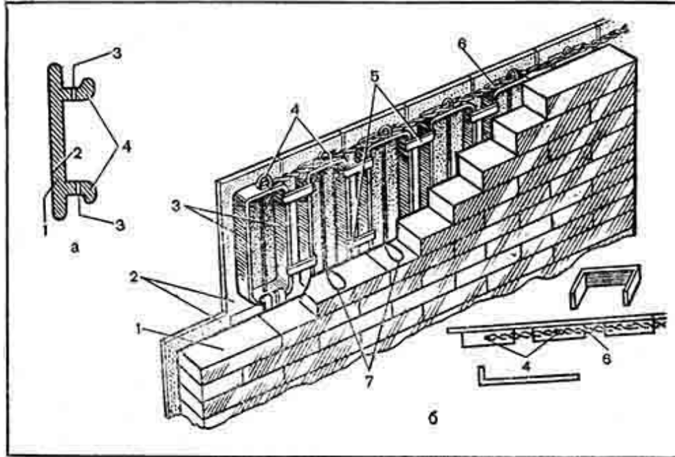
Рис. 94. Облицовка печи изразцами:
