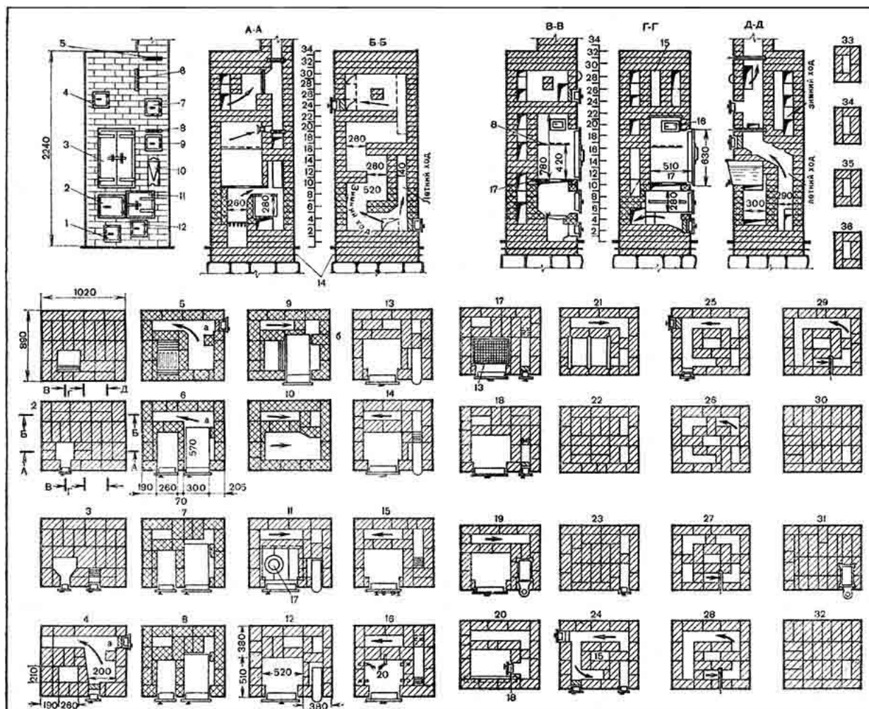
Рис. 65. Отопительно-варочная печь конструкции И. Ф. Волкова:
