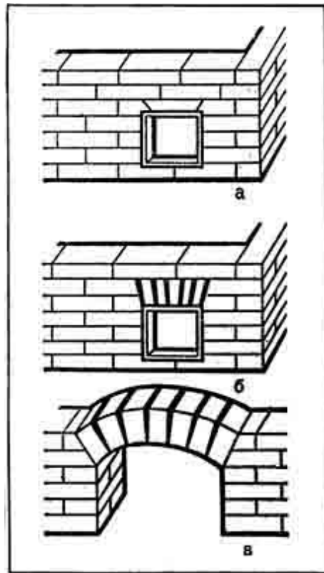
Рис. 30. Перекрытие проемов печей и топливников над топочными дверками:
