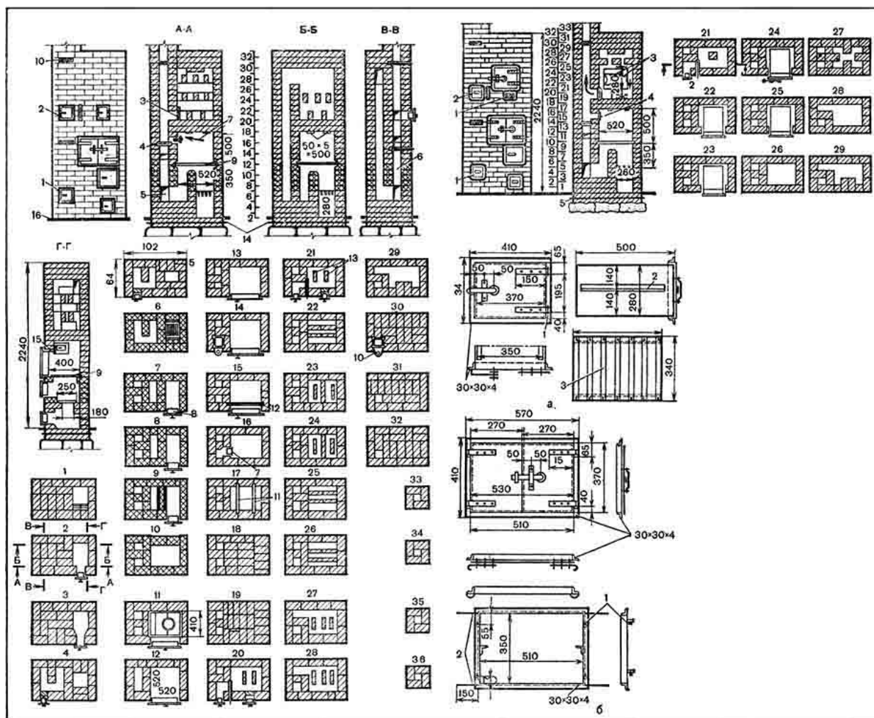
Рис. 64. Отопительно-варочная печь обычная и с тепловым шкафом:
