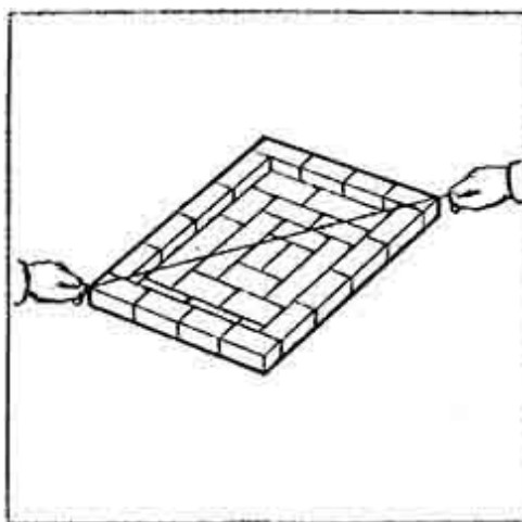
Рис. 13. Проверка закладки первого ряда кладки печи
