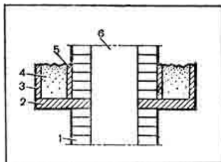
Рис. 91. Изготовление распушки с заполнителем:
