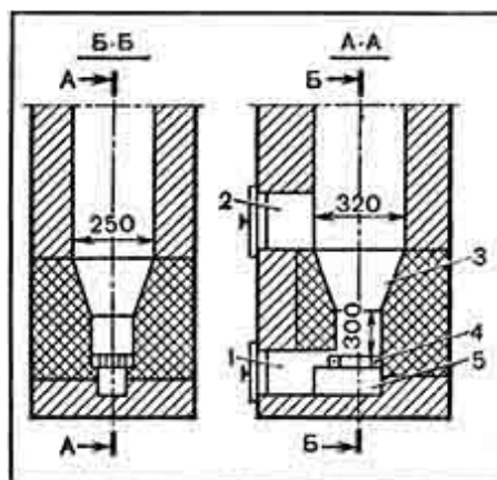
Рис. 42. Топливник для каменного угля:
