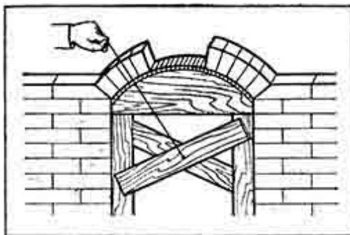
Рис. 35. Проверка правильного расположения швов кладки в арке
