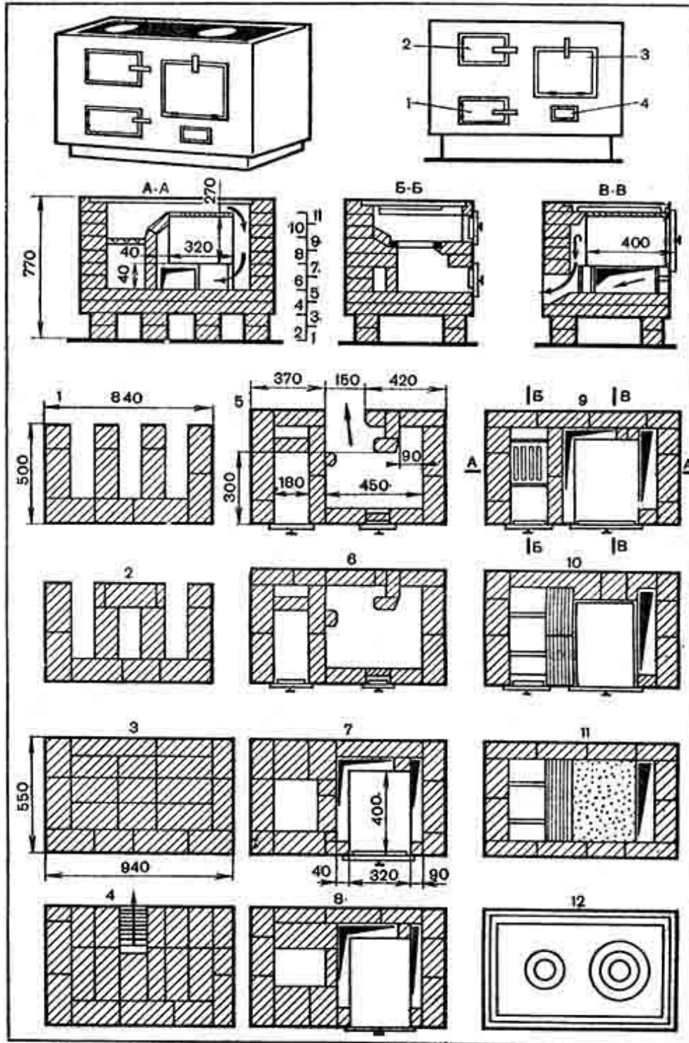
Рис. 51. Кухонная плита на шанцах с духовкой, равномерно обогреваемой со всех сторон: 1 — поддувало; 2 — топливник; 3 — духовка; 4 — чистка
