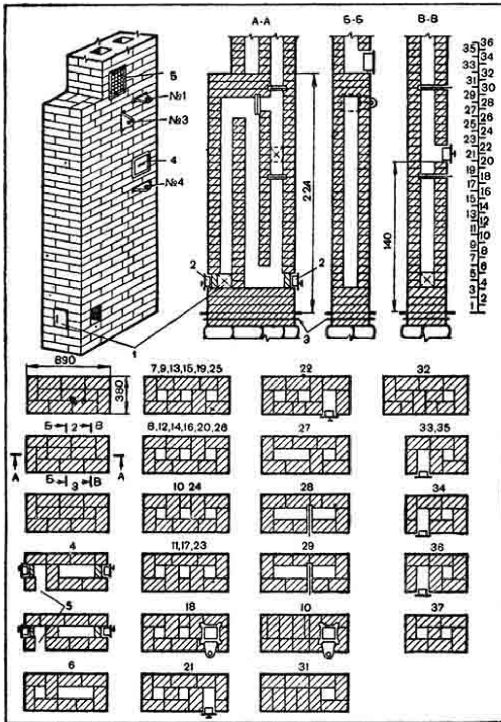
Рис. 59. Отопительный щиток толстостенный:
