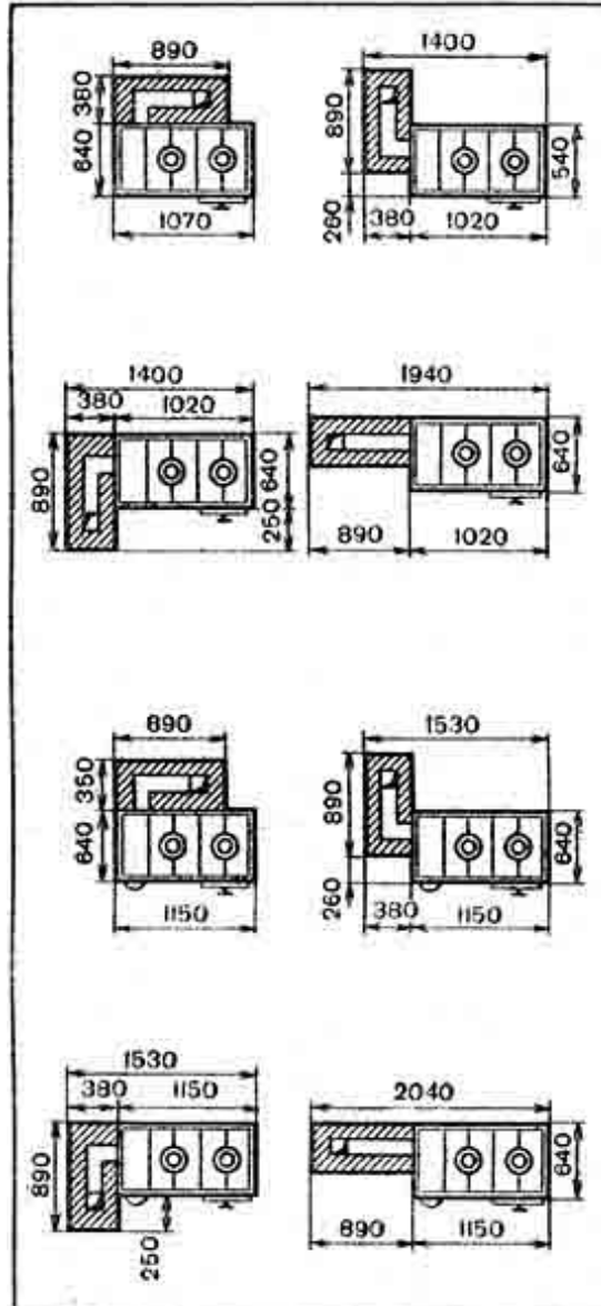
Рис. 54. Схемы присоединения плиты к отопительным щиткам
