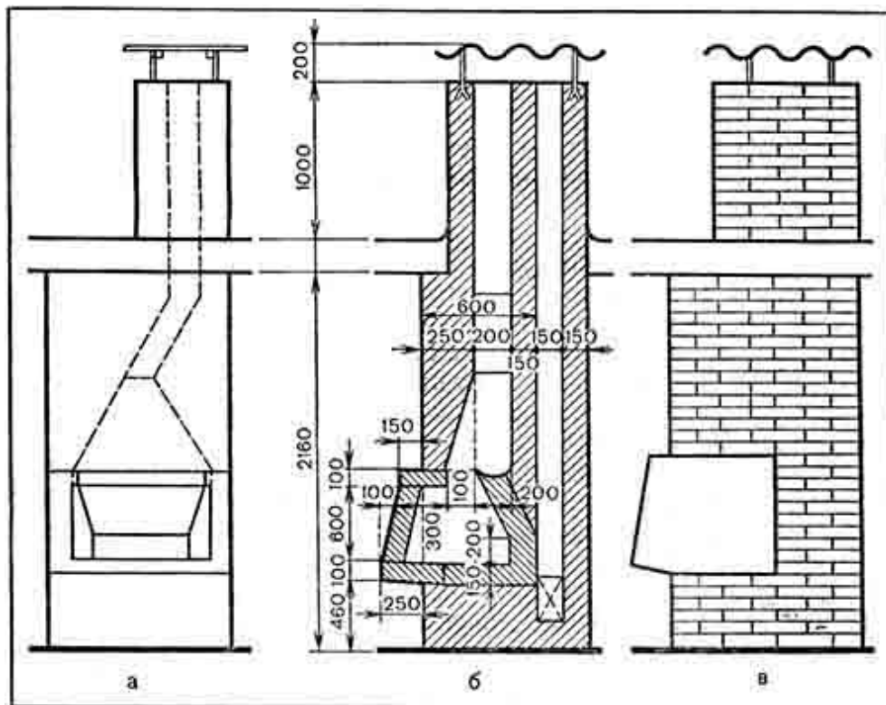
Рис. 108. Камин из кирпича: a — вид спереди; б — разрез; в — вид сбоку
