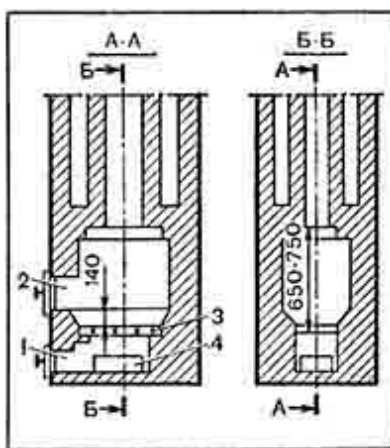
Рис. 40. Топливник для торфа:
