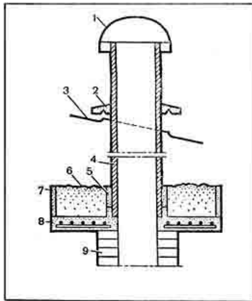
Рис. 93. Асбестоцементная труба:
