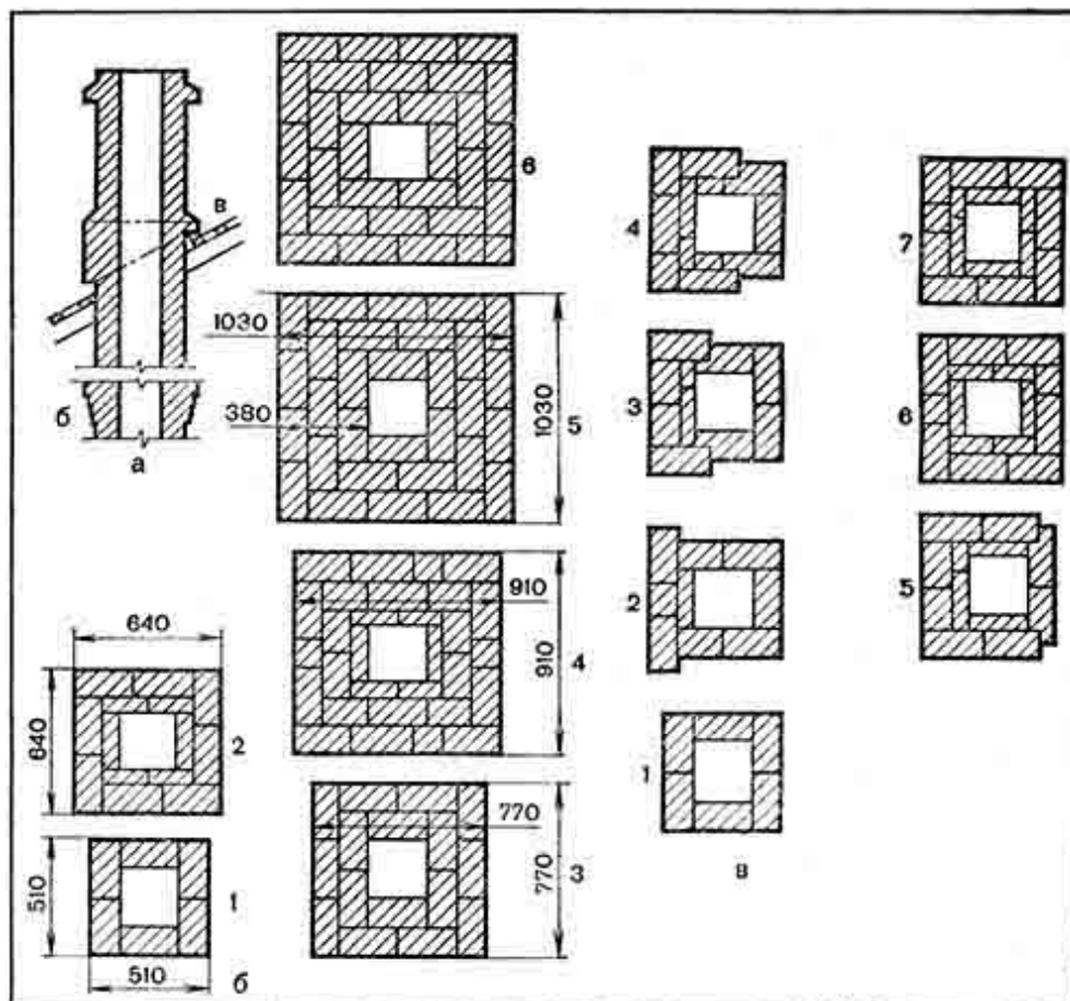
Рис. 89. Кладка распушки и выдры с дымовым каналом 27x27 см: a — общий вид трубы; б — порядовки распушки; в — порядовки выдры
