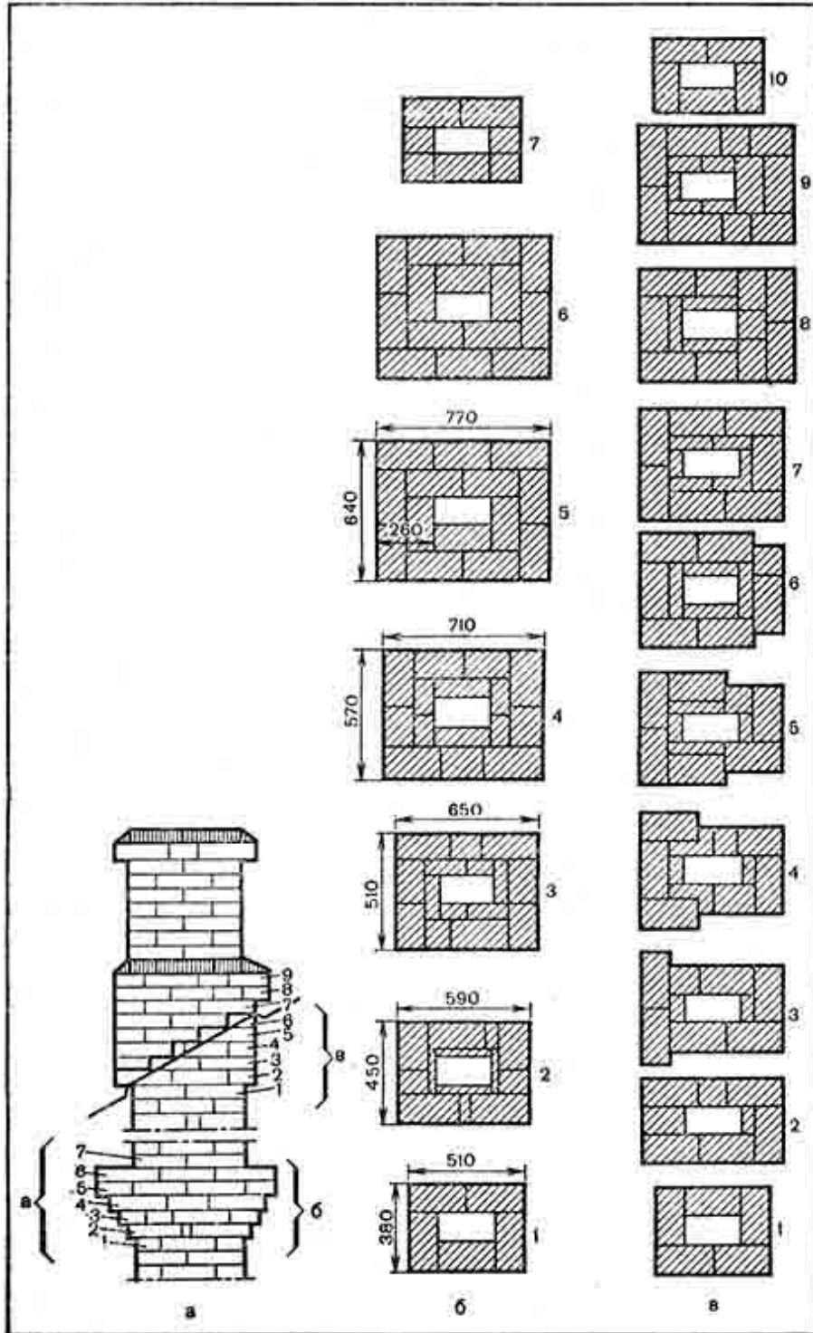
Рис. 88. Кладка распушки и выдры с дымовым каналом 14x27 см: a — общий вид трубы; б — порядовки распушки; в — порядовки выдры
