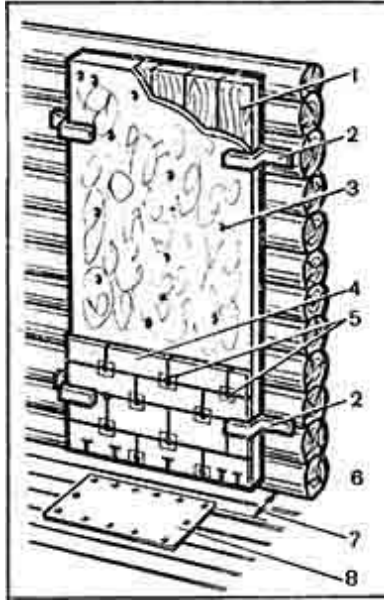
Рис. 95. Изоляция стен от печи:
