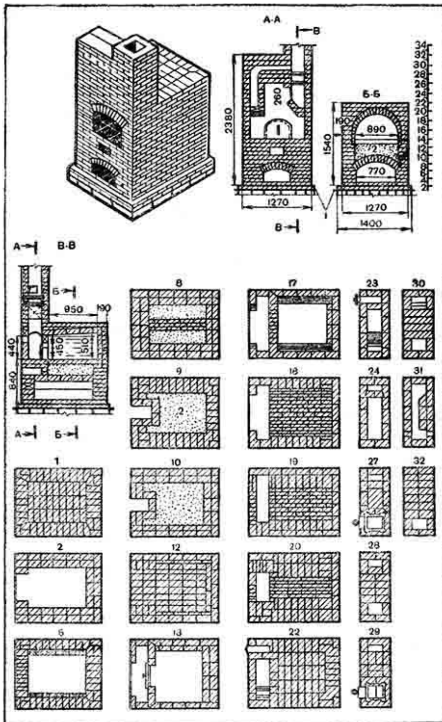
Рис. 69. Русская обыкновенная печь:
