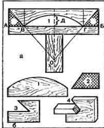
Рис. 32. Построение кружала для свода и шаблона для пята: a — построение кружала; б — кружало и шаблоны; 1 — кружало; 2 — шаблон пята; 3 — шаблон для тески пята; 4 — проверка отесанного кирпича
