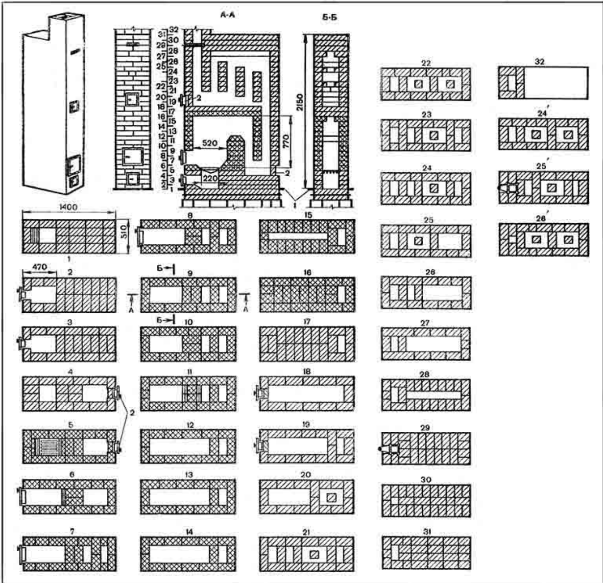
Рис. 76. Отопительная печь, оштукатуренная, с теплоотдачей 2400 ккал/ч:
