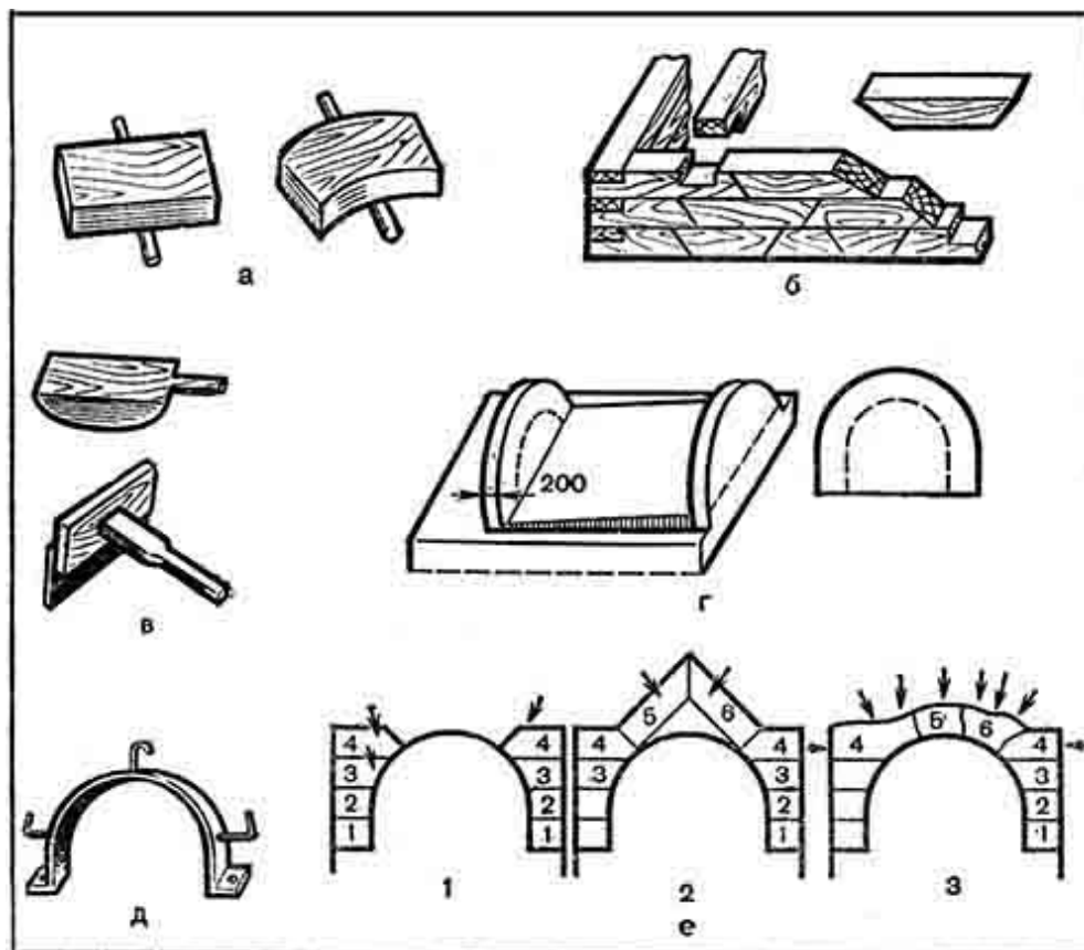
Рис. 73. Приспособление и порядок устройства русской глинобитной печи:
