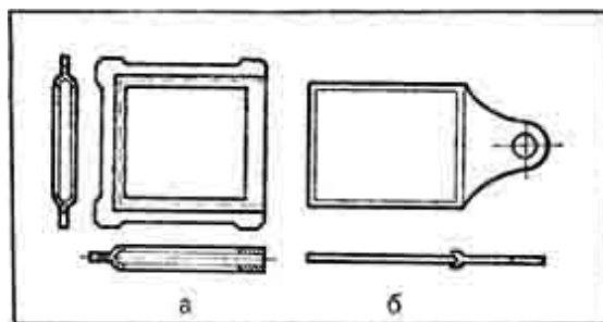
Рис. 8. Задвижка печная:
