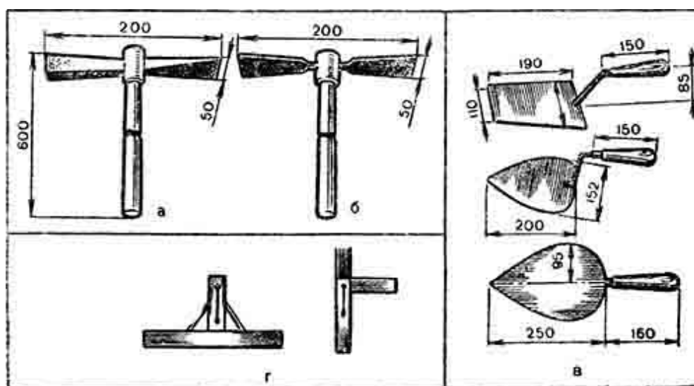
Рис. 11. Инструменты для печных работ: а — печной молоток; б — кирочка; в — кельма; г — ватерпас
