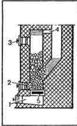
Рис. 43. Топливник шахтный для каменного угля:
