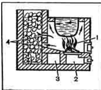
Рис. 113. Печь-каменка с поддувалом:
