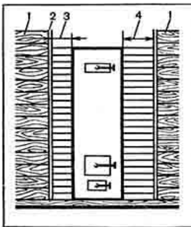
Рис. 97. Отступка между печью и деревянными перегородками:
