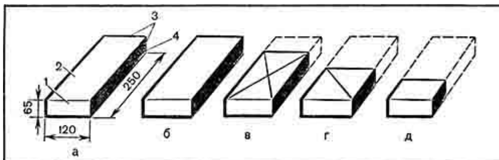
Рис. 16. Кирпич и его части:
