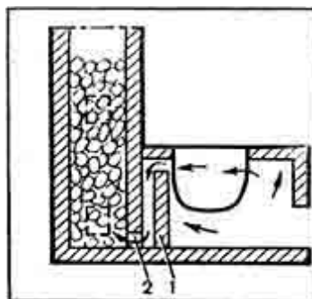
Рис. 112. Улучшенная печь-каменка со стенкой для направления горячих газов: 1 — стенка внутри топливника; 2 — отверстие в стенке камеры
