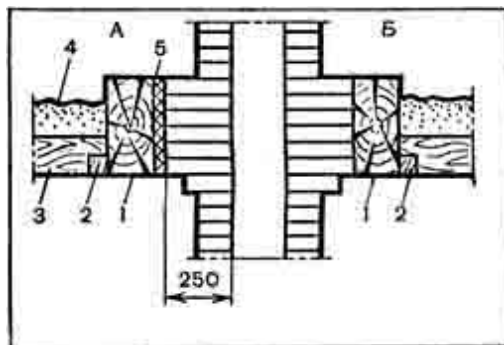
Рис. 100. Разделка распушки в чердачном перекрытии:
