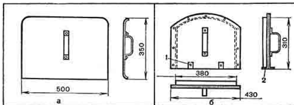
Рис. 10. Заслонки:
