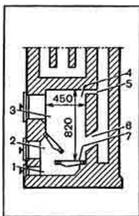
Рис. 41. Топливник для торфа повышенной влажности:
