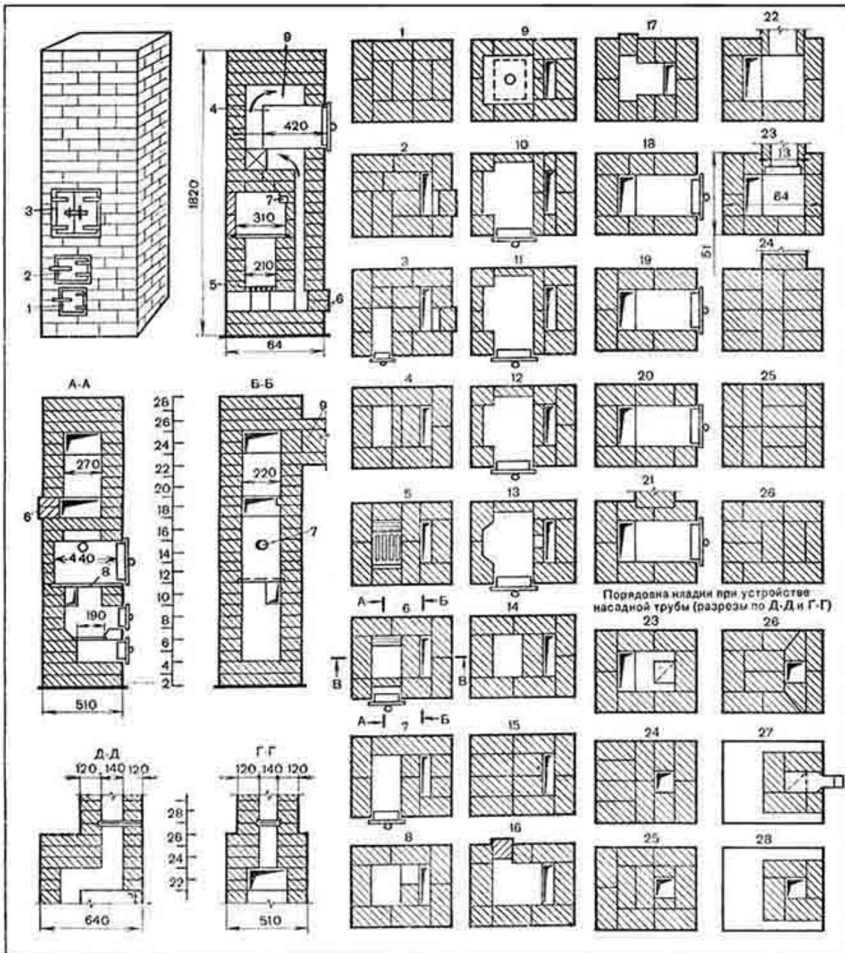
Рис. 62. Отопительно-варочная печь конструкции В. А. Потапова (первый вариант):
