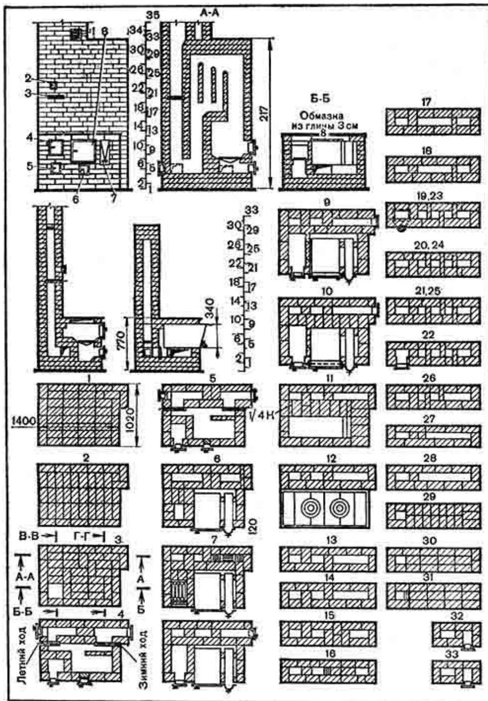
Рис. 61. Кухонная плита со щитком, имеющим самостоятельную топку:
