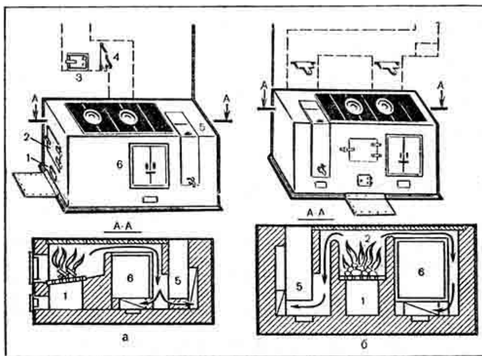
Рис. 48. Кухонные плиты:
