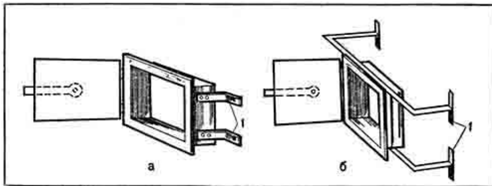
Рис. 7. Крепление лапок к рамкам дверок: а — лапки простые; б — улучшенные; 1 — лапки
