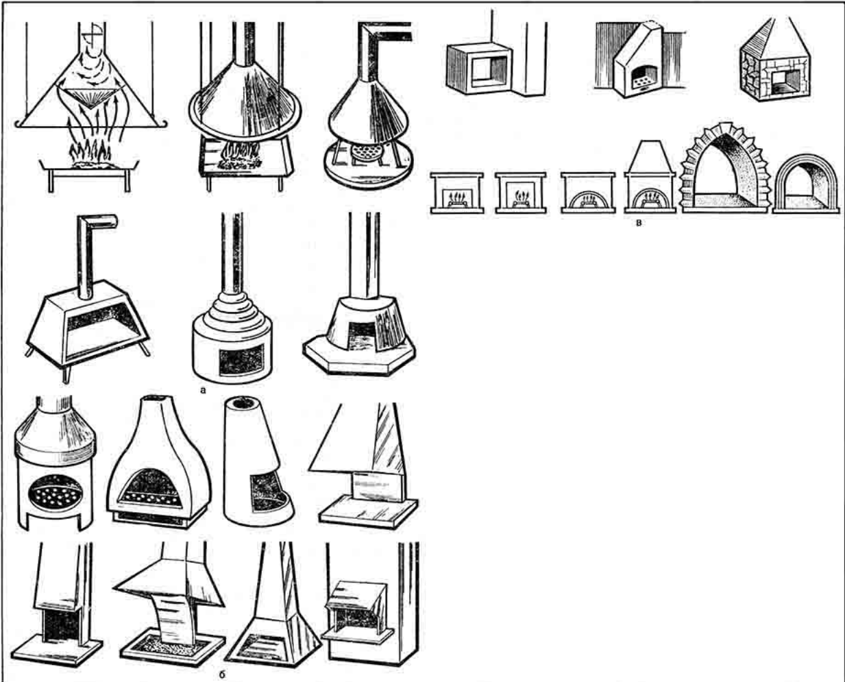
Рис. 106. Разновидности каминов:
