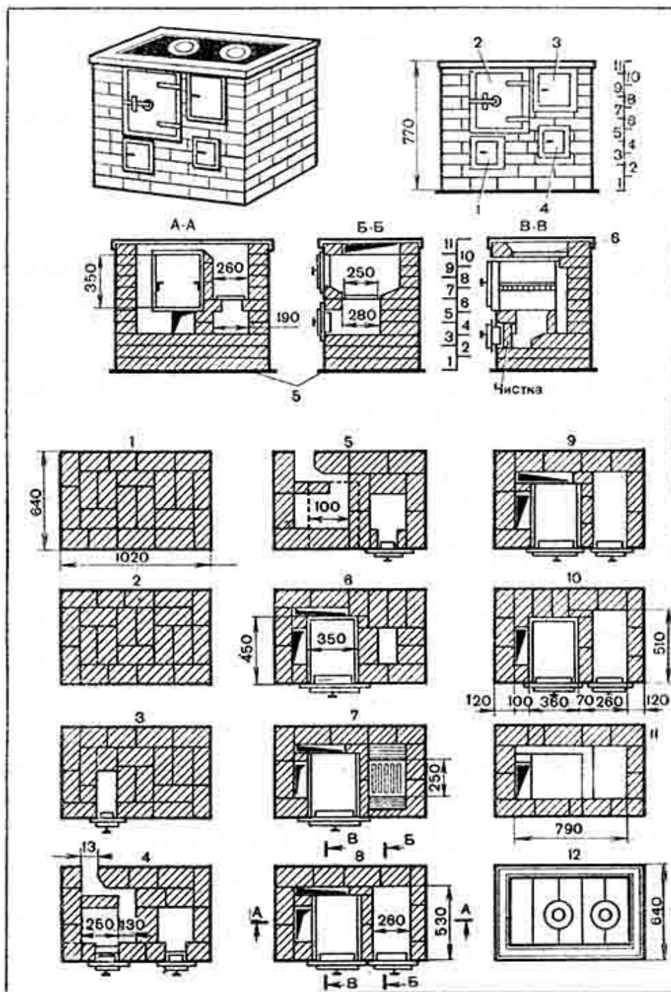
Рис. 50. Кухонная плита с духовкой:
