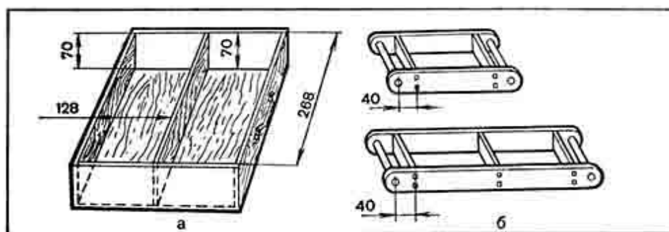
Рис. 3. Формы для изготовления кирпича:
