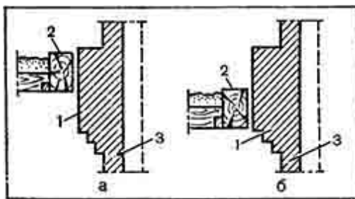
Рис. 102. Расположение распушки с учетом осадки перекрытия: а — до осадки; б — после осадки; 1 — распушка; 2 — перекрытие; 3 — стояк трубы
