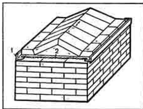
Рис. 28. Укрепление пят треугольного свода путем сжатия угловой или полосовой сталью со стягиванием проволочным жгутом:
