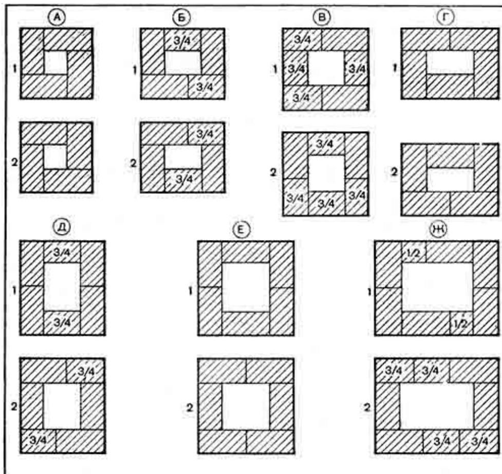
Рис. 85. Размеры дымовых каналов и их кладка: 1 — нечетные ряды; 2 — четные ряды
