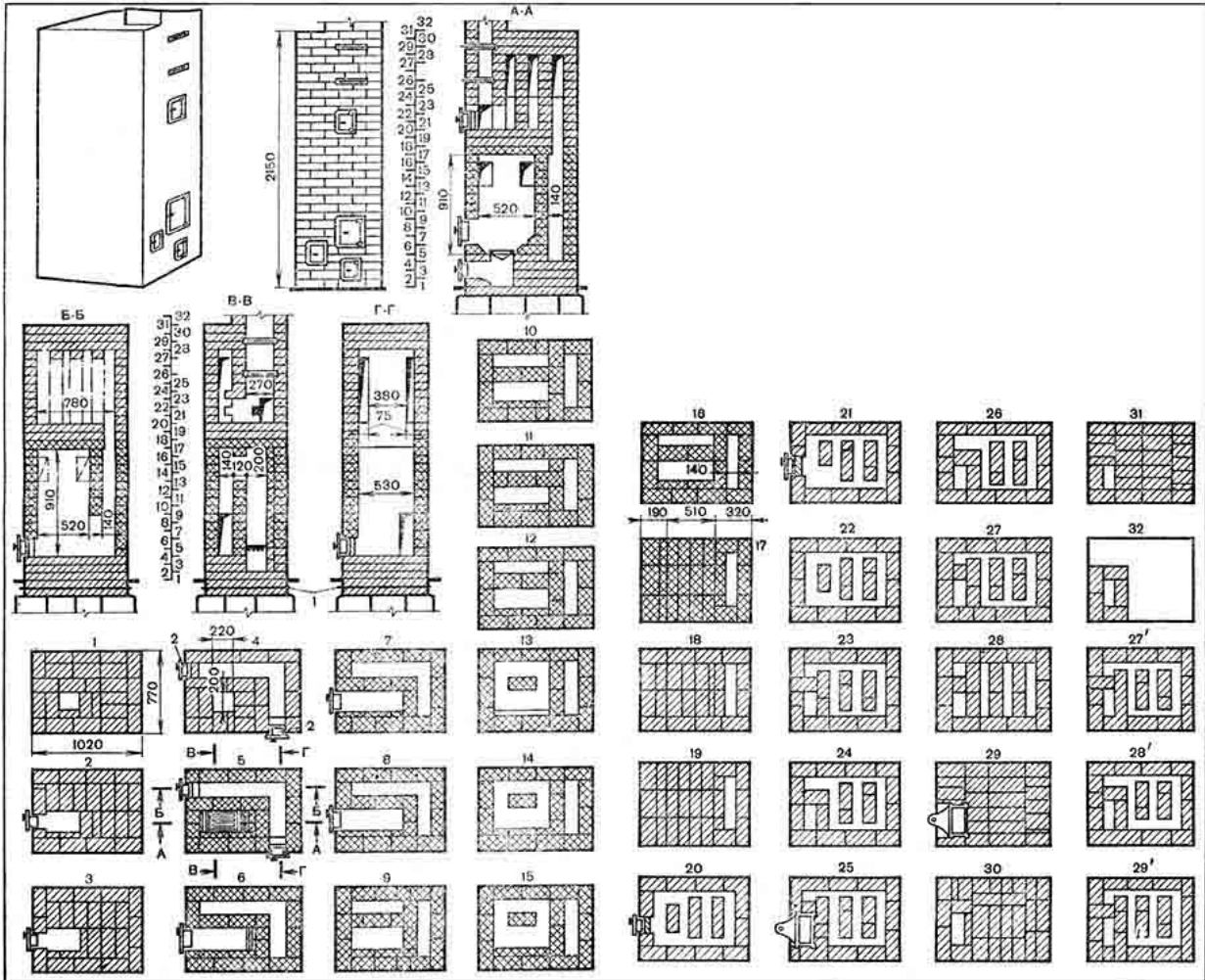
Рис. 77. Отопительная печь, оштукатуренная, с теплоотдачей 3020 ккал/ч:
