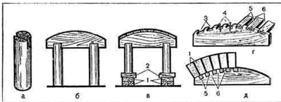
Рис. 34. Устройство разъемной опалубки:
