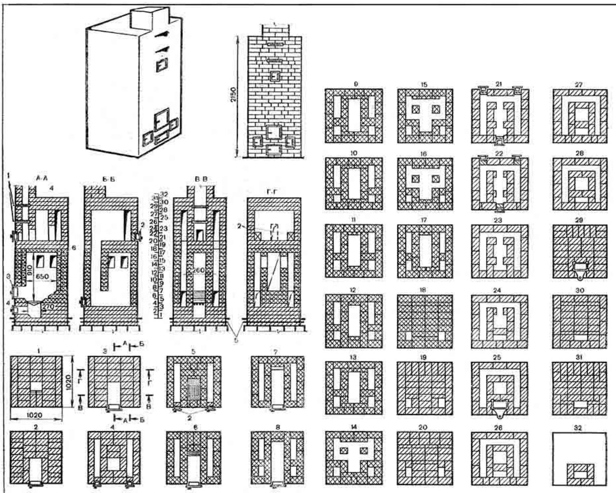
Рис. 78. Отопительная печь, оштукатуренная, с теплоотдачей 3850 ккал/ч:
