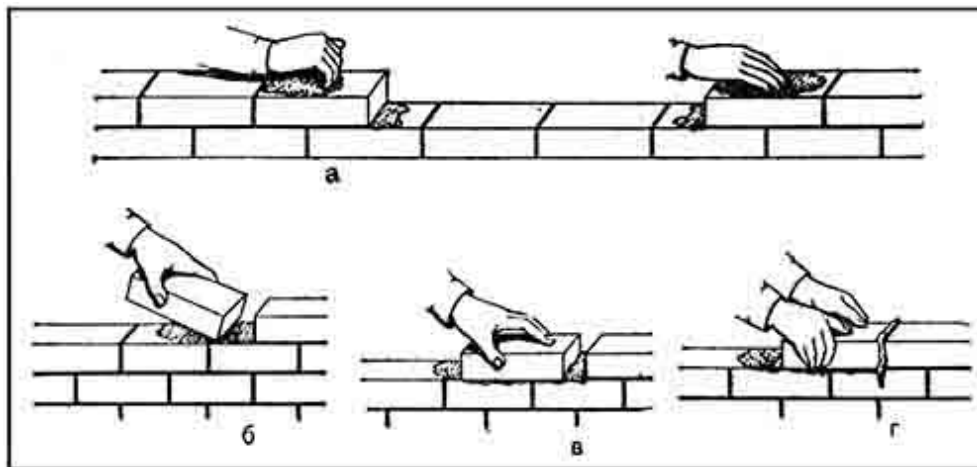
Рис. 24. Укладка кирпича на раствор:
