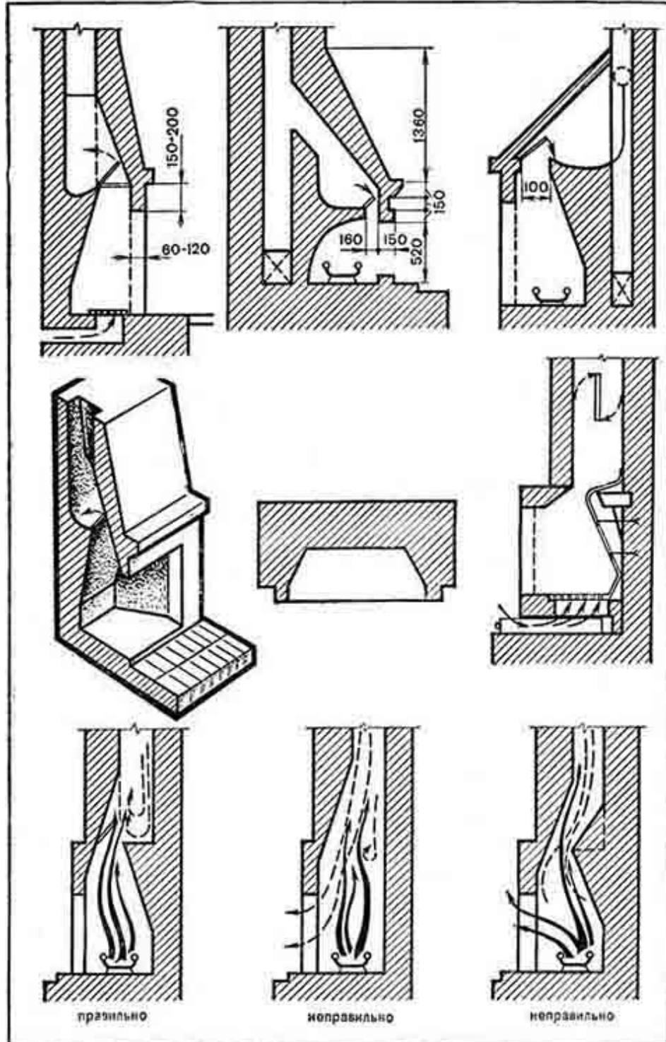
Рис. 105. Разрезы каминов и форма газовых порогов
