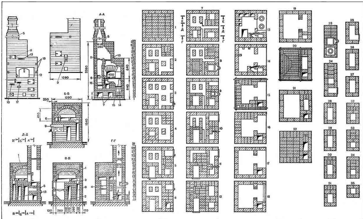
Рис. 72. Улучшенная русская печь «Теплушка» с плитой конструкции И. С. Подгородникова:
