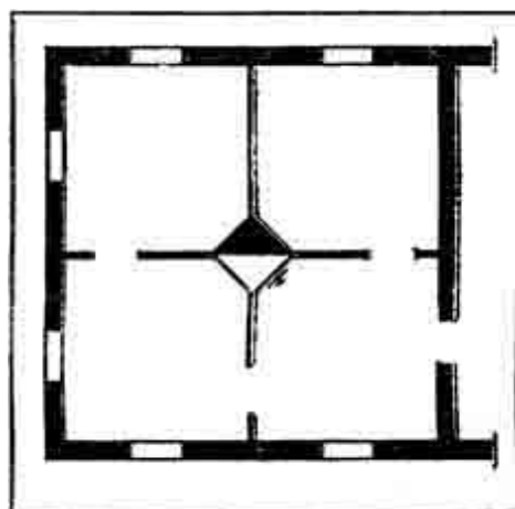
Рис. 20. Установка одной печи для отапливания четырех комнат
