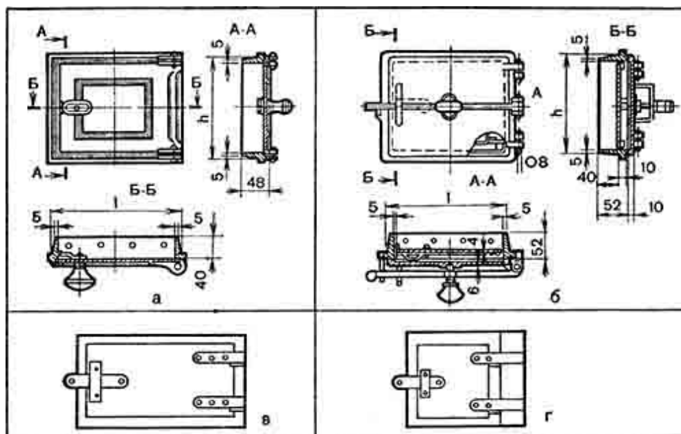
Рис. 5. Дверки и полудверки:
