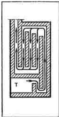
Рис. 47. Схема с преимущественным нижним прогревом:
