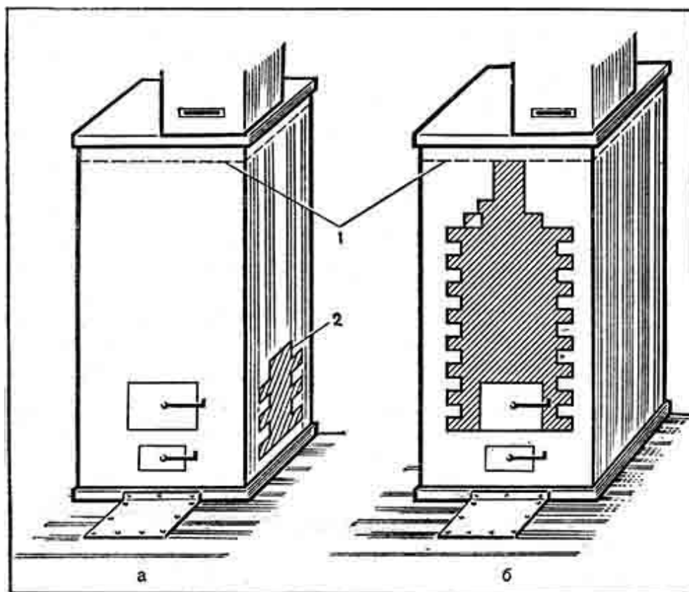
Рис. 103. Ремонт печей:
