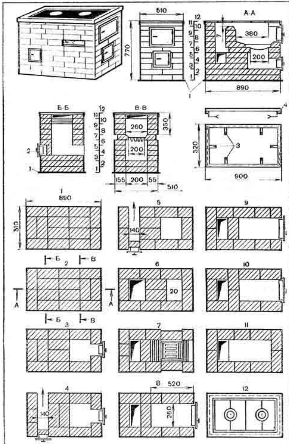
Рис. 49. Кухонная плита упрощенная:
