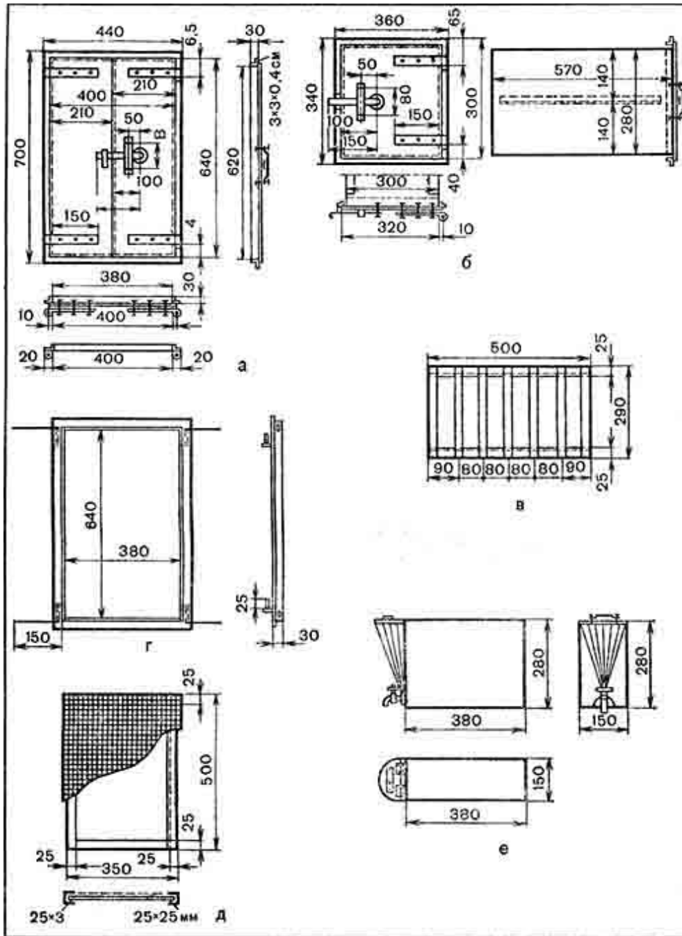
Рис. 66. Изготовление дверок, решеток, водогрейной коробки для отопительно-варочной печи:
