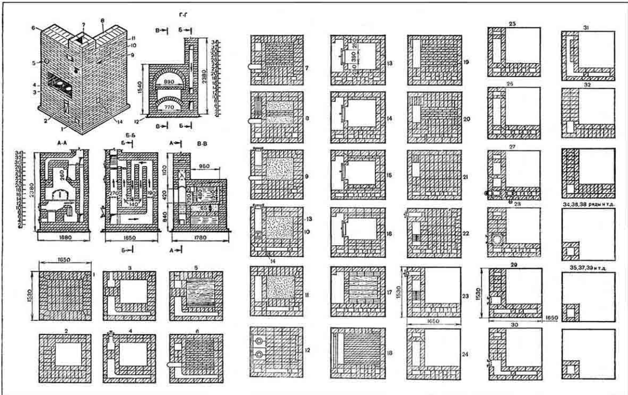
Рис. 71. Русская печь с плитой и обогревательным щитком:
