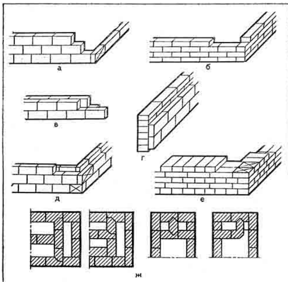
Рис. 18. Печная кладка стенок разной толщины:
