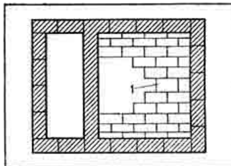
Рис. 36. Кладка свода отдельными захватками:
