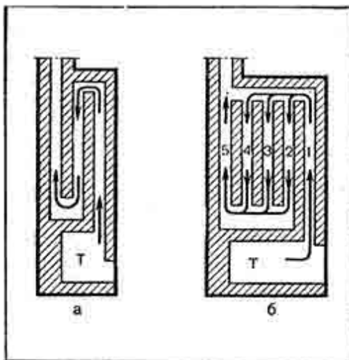
Рис. 44. Малооборотные схемы:
