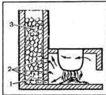
Рис. 111. Улучшенная печь-каменка: 1, 3 — дверки; 2 — отверстие в стенке топливника
