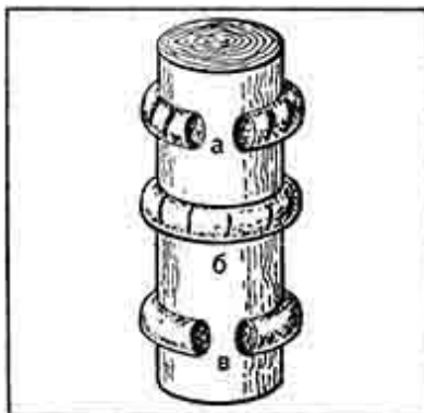
Рис. 2. Проверка на сгибание жгутиков из глиняного раствора: а — тощего; б — нормального; в — жирного
