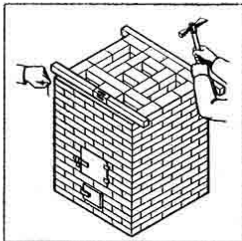
Рис. 14. Проверка выполненной печной кладки
