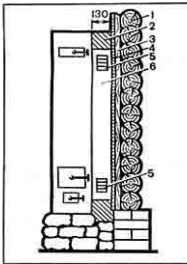
Рис. 96. Отступка между печью и деревянной стеной:
