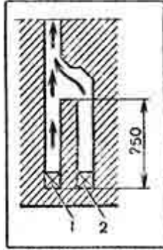
Рис. 82. Присоединение двух печей к одному дымоходу:
