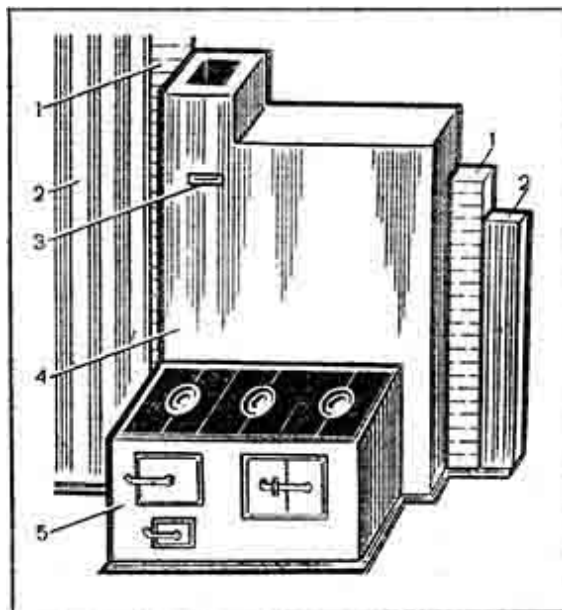
Рис. 56. Кухонная плита с постоянно нагреваемым отопительным щитком:
